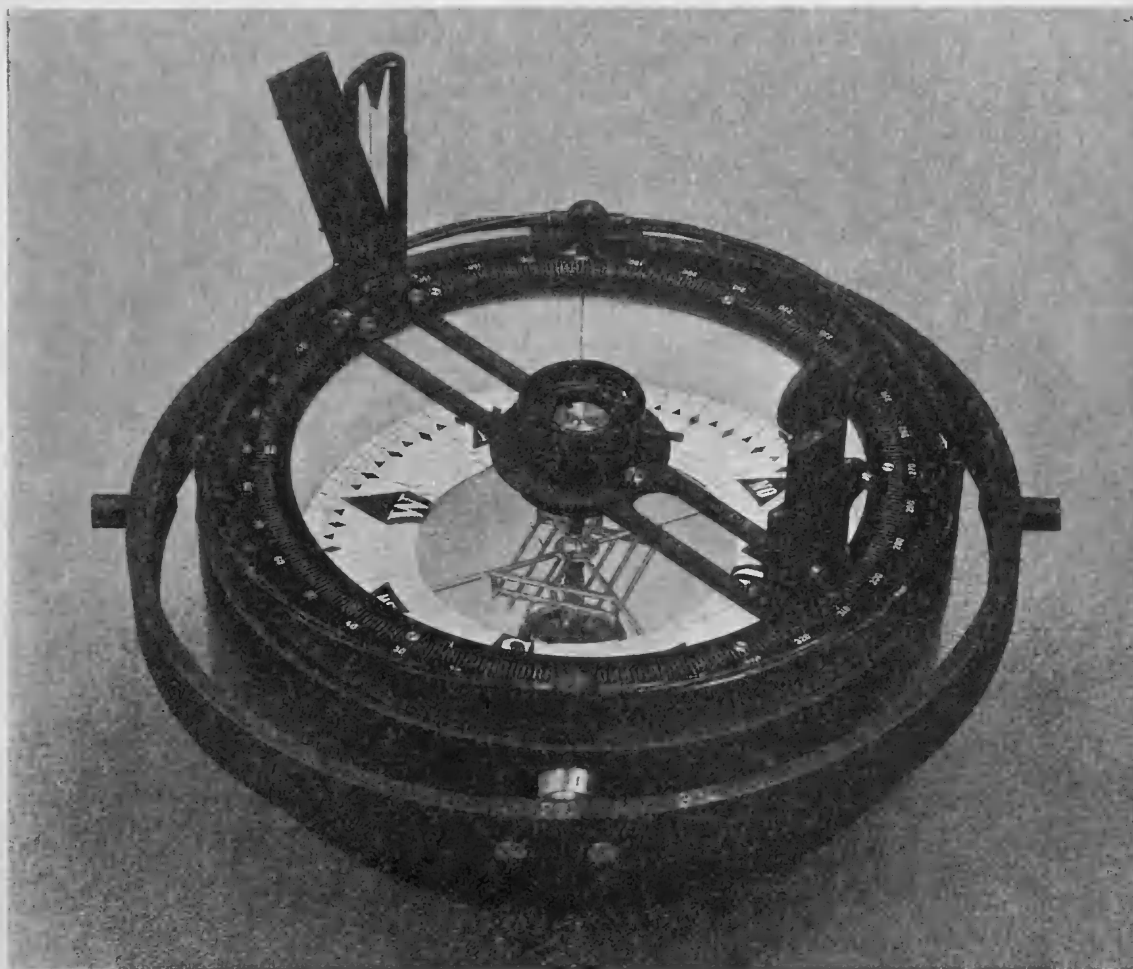
1. Видъ компаснаго котелка сверху, съ картушкой, азимутальнымъ кругомъ, алидадой и подвѣсомъ.
